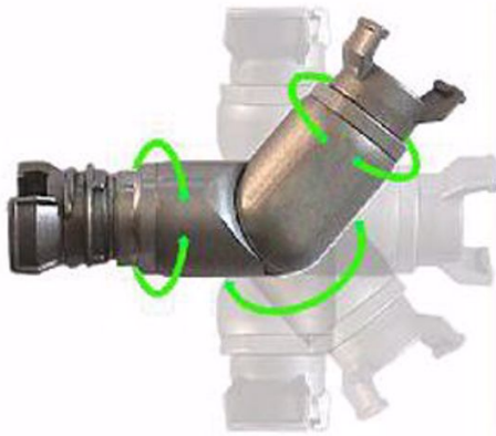
Claw couplers optional extra
